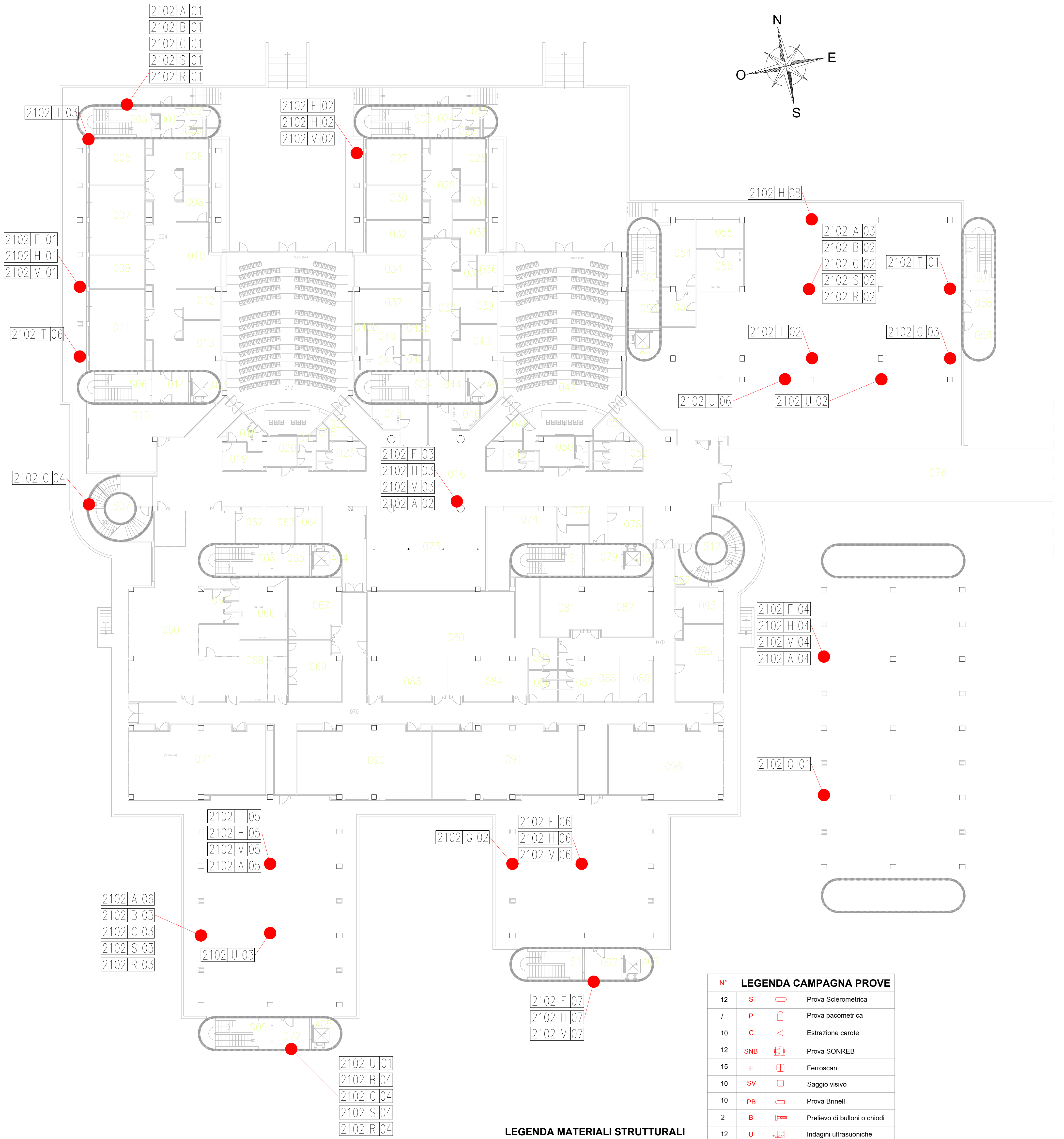
PIANTA PIANO SEMINTERRATO Scala 1:200
