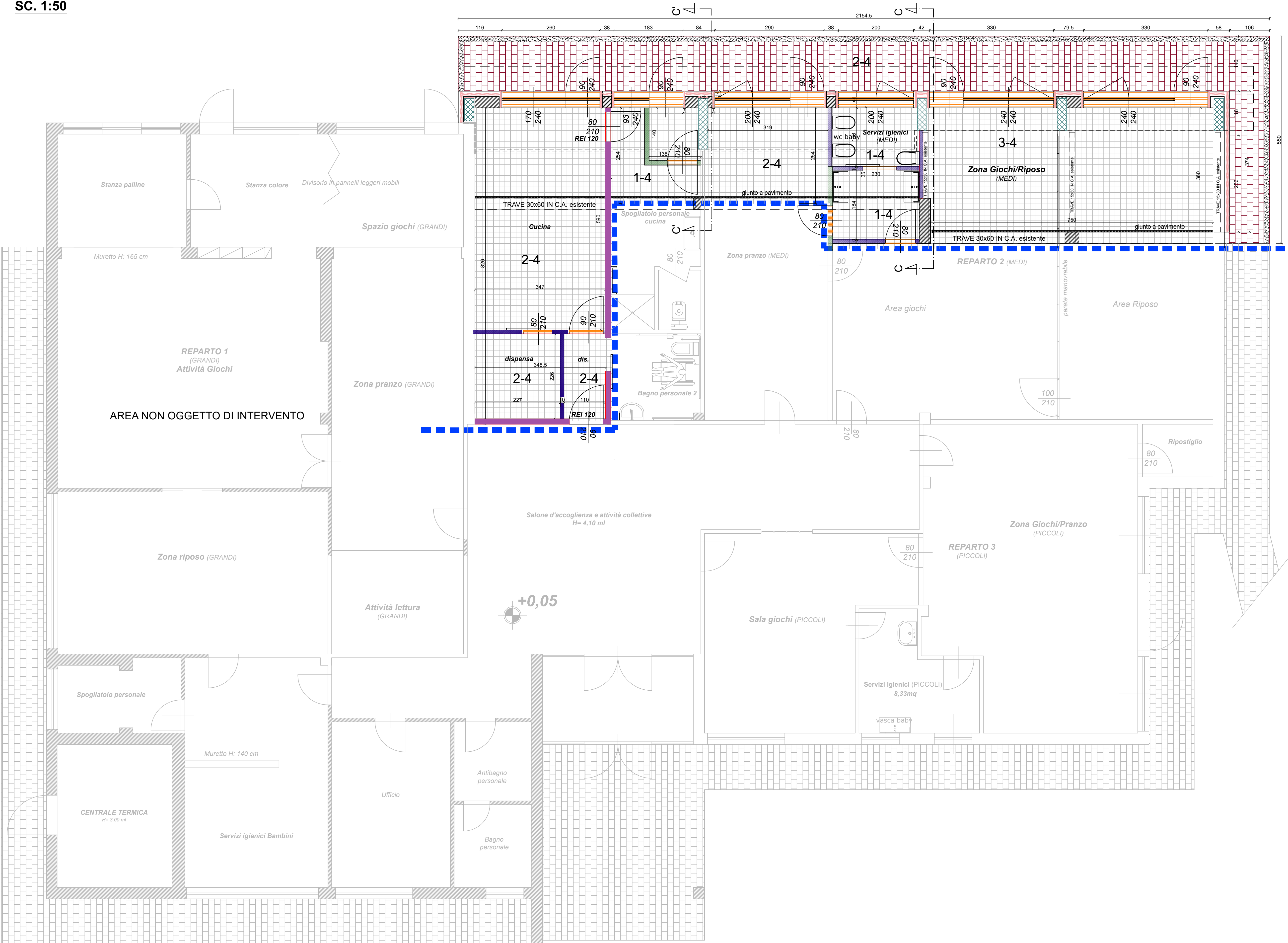
PIANTA PIANO TERRA STATO DI PROGETTO - SC. 1:50
