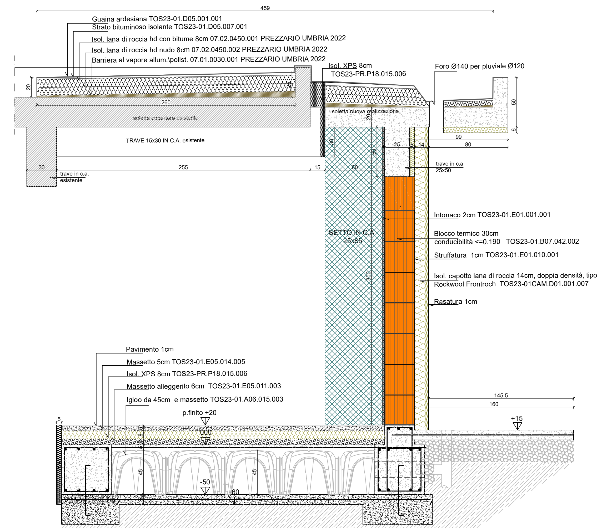
SEZIONE C'-C' Sc.1:20
