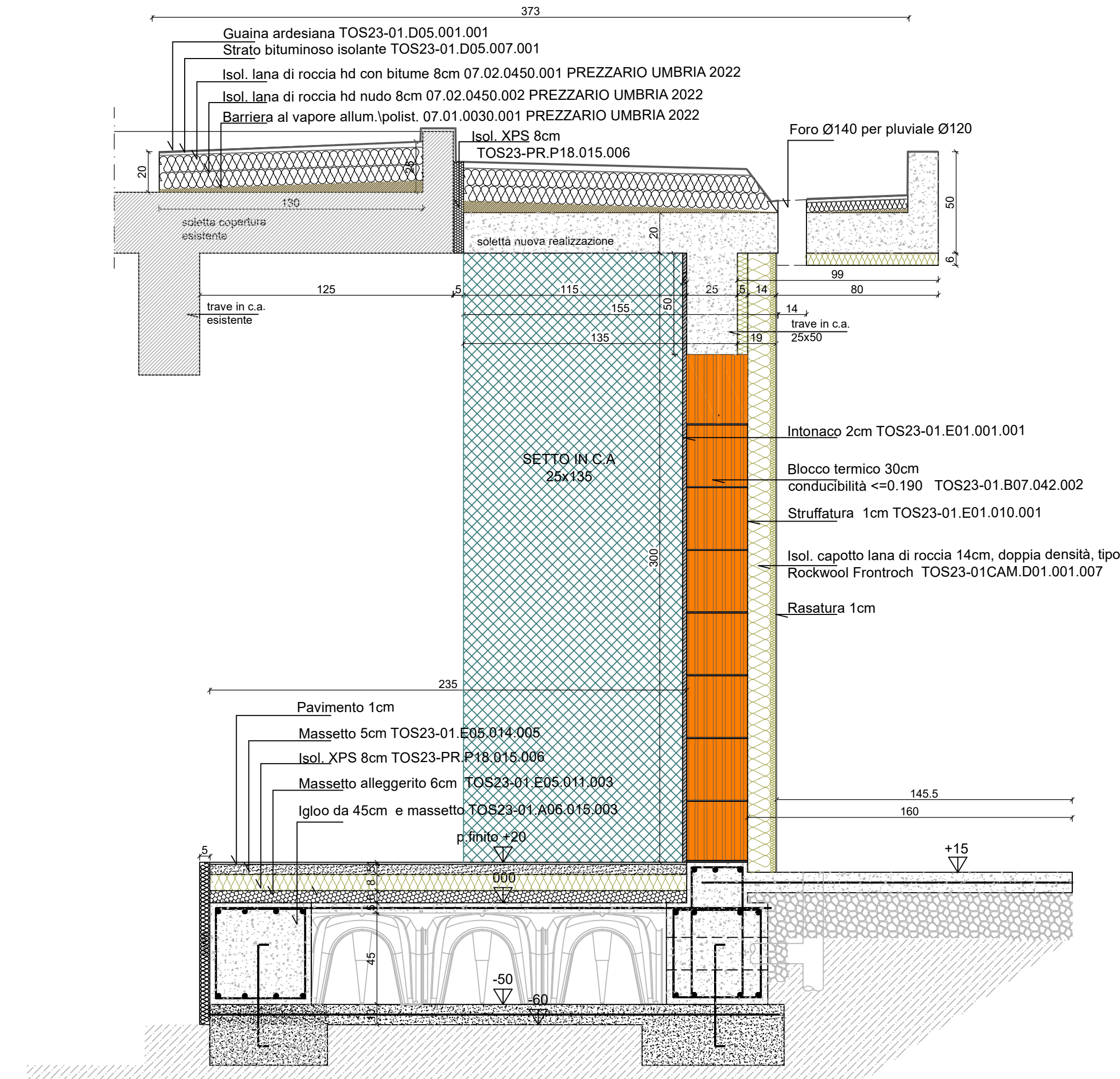
SEZIONE C'-C' Sc.1:20
